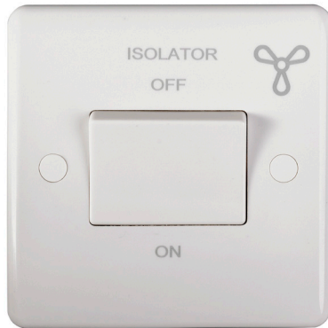
10A 3 POLE FAN ISOLATOR SWITCH 86x86x7mm
